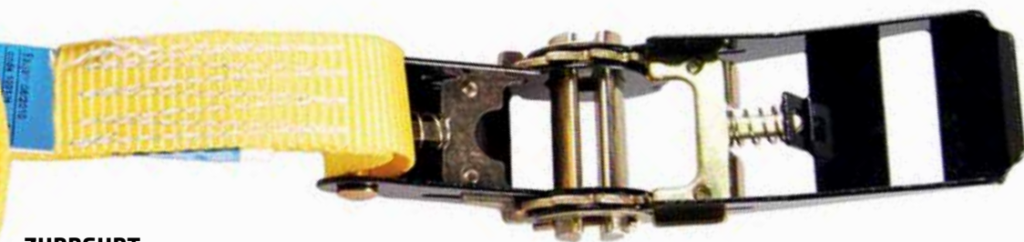
ZURRGURT mit Ratsche, Länge 6 m, Breite 25 mm, LC 800 daN, 1-teilig Art.-Nr. 40530
